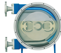
蠕动（软管）泵
